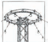
DÉTAIL TRUSS + CERCE
